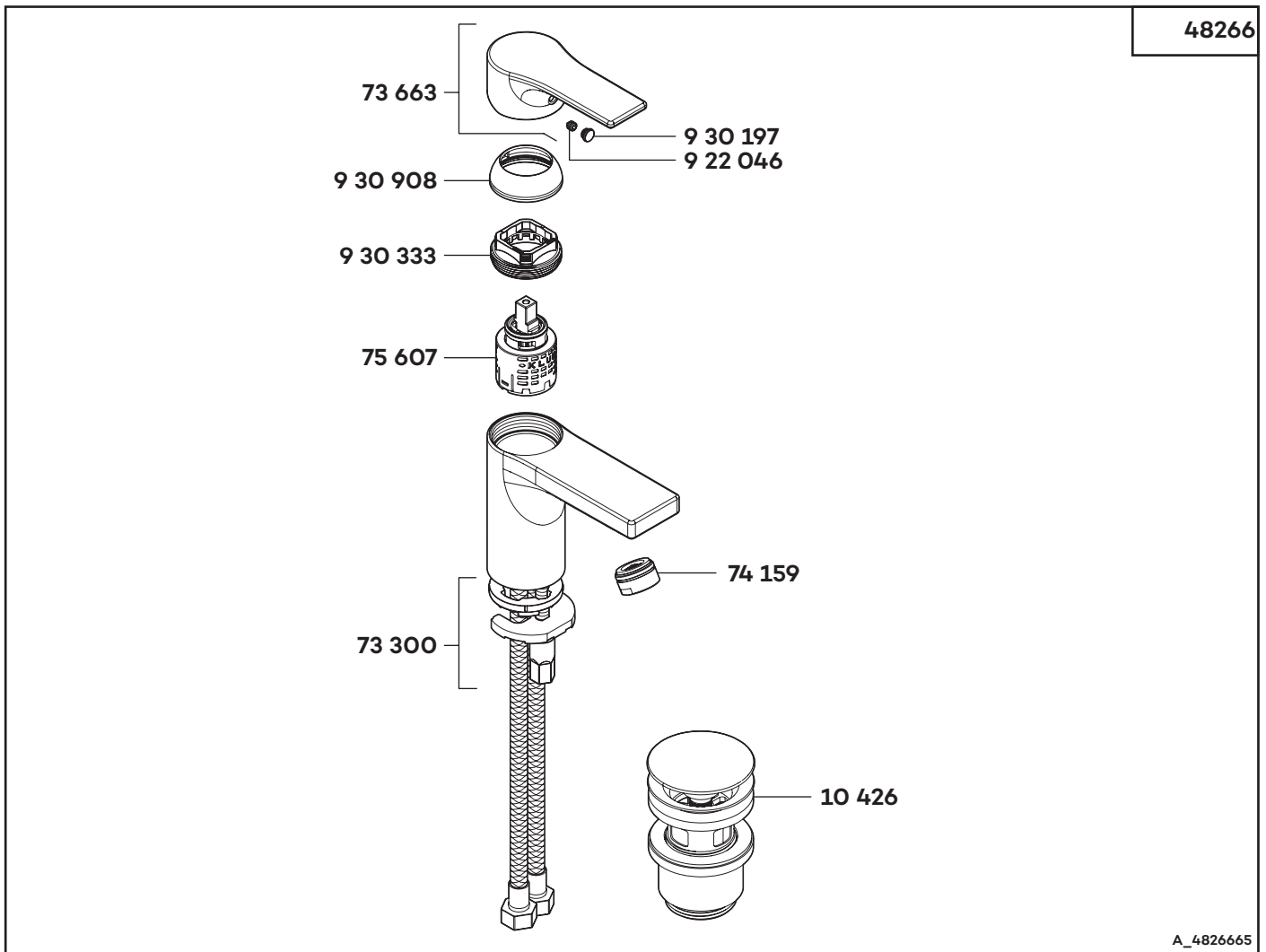
48266 Waschtisch-Einhandmischer DN 15 single lever basin mixer DN 15 ééngreeps wastafelmengkraan 1/2"
